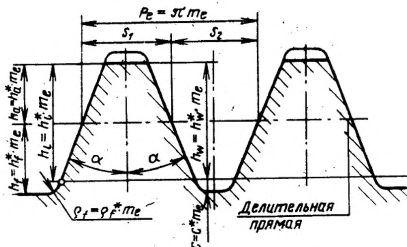
Пара исходных контуров
