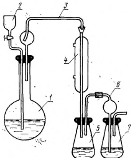
1—перегонная колба; 2—канальная воронка; 3—насадка с брызгоулавливателем; 4—холодильник; 5—приемник, 6—отводная трубка с шариком; 7—контрольный приемник
