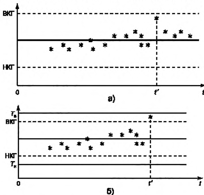
Рисунок А.1 — Контрольная карта Шухарта (а) и приемочная контрольная карта средних арифметических значений мгновенных выборок (б) в момент времени t'
