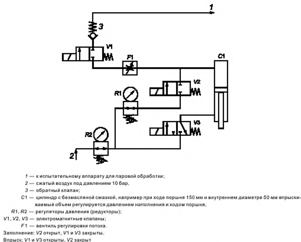
Рисунок L.1 — Примерная схема системы впрыска воздуха
