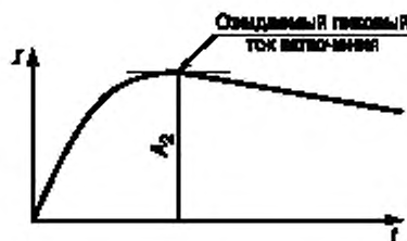
Рисунок 7b — Калибровка испытательной цепи для постоянного тока
