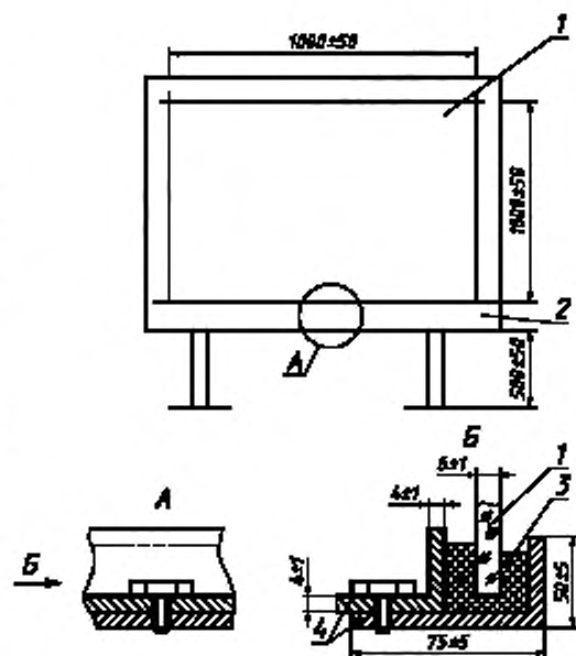
1 — стеклянный лист; 2 — станина; 3 — резиновая прокладка; 4 — монтажные уголки
