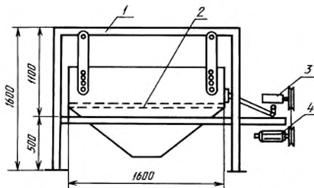
1 — рама; 2 — сетка размером 1200 × 1600 мм с отверстиями 12 × 12 или 25 × 25 мм; 3 — редуктор; 4 — электродвигатель
