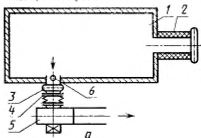
Измерение шума нагнетания
