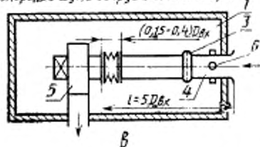
Измерение шума вокруг вентилятора
