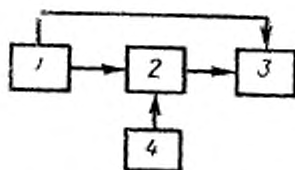
1—источник импульсов излучения с ослабителем потока излучения; 2—светонепроницаемая камера с фотоумножителем; 3—источник питания фотоумножителя с делителем напряжения (или отдельные источники питания электродов) и вольтметром контроля режима; 4—осциллограф
