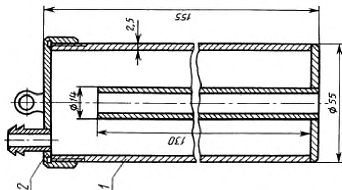
Металлический переносный проботборник
