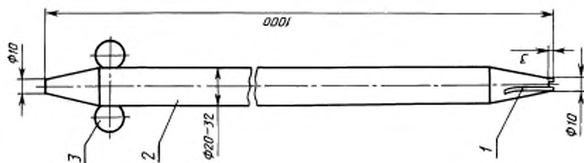
Пробоотборная трубка
