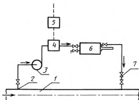
Схема отбора проб из трубопровода с применением пробоотборника с выравненным давлением
