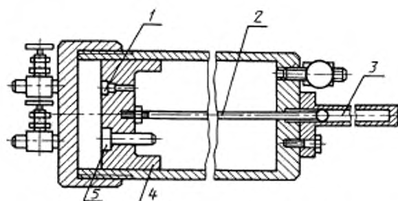
Пробоотборник с выравненным давлением
