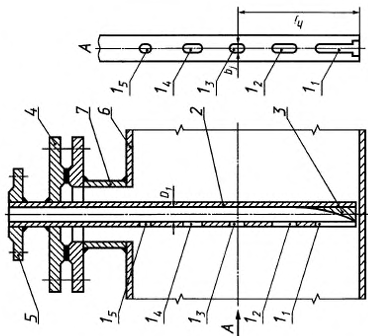
1 1 — 1 5 — отверстия; 2 — трубка; 3 — стабилизатор; 4 — крышка; 5 — штанг; 6 — трубопровод; 7 — монтажный патрубок
