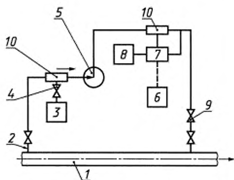
Схема отбора проб нефти из трубопровода при помощи пробозаборных устройств щелевого типа
