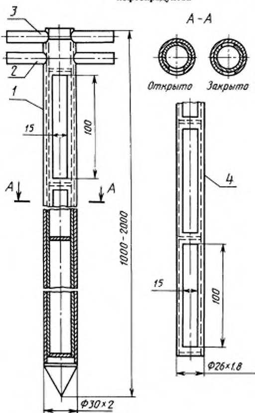
Щуп для отбора проб порошкообразных нефтепродуктов
