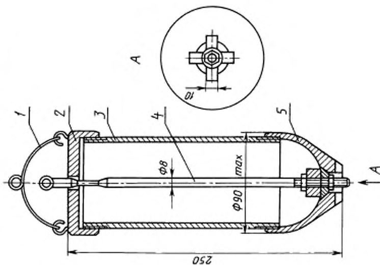
Металлический переносный пробоотборник
