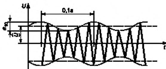
Рисунок 6 — Синусоидальная модуляция напряжения амплитудой 0,1 и регулярной частотой 10 Гц
