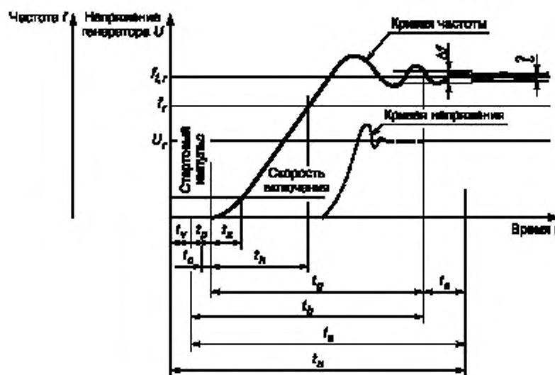
Рисунок 10 — Пусковые характеристики
