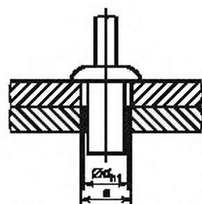
Рисунок 2 — Увеличенный диаметр отверстий для облегчения совмещения
