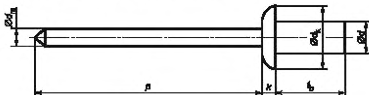
Рисунок 1 — Размеры заклепок
