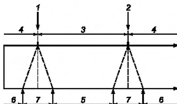
1 — нижний предел требований; 2 — верхний предел требований; 3 — зона требований (поле допуска); 4 — выход за пределы требований; 5 — зона соответствия; 6 — зона несоответствия; 7 — погрешность измерений
