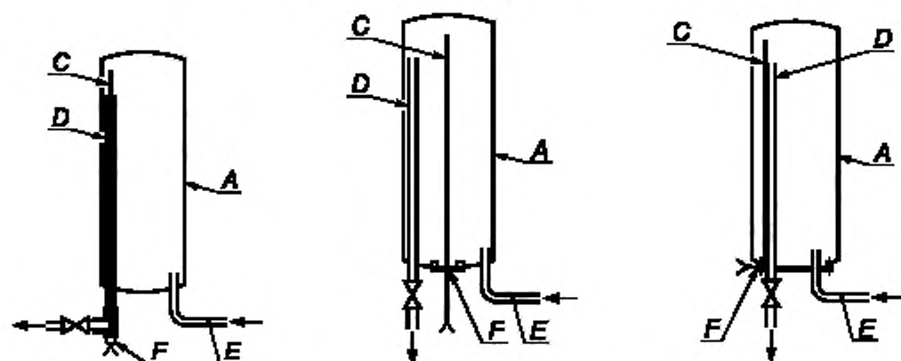
а — Положение термодпар для металлических баков
