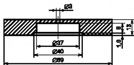
Рисунок 2 — Монтажный блок калориметра
