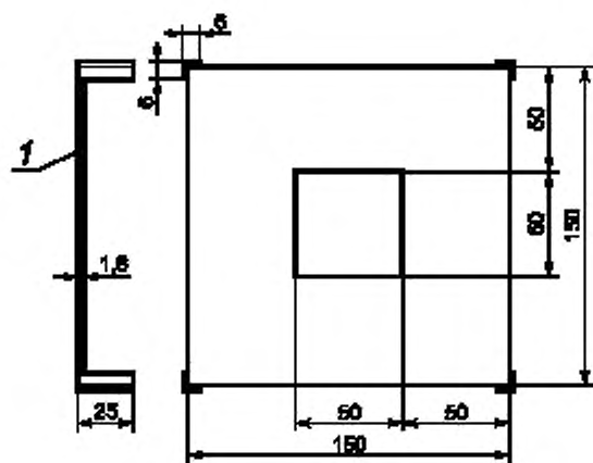
Рисунок 3 — Опорная рама для образца
