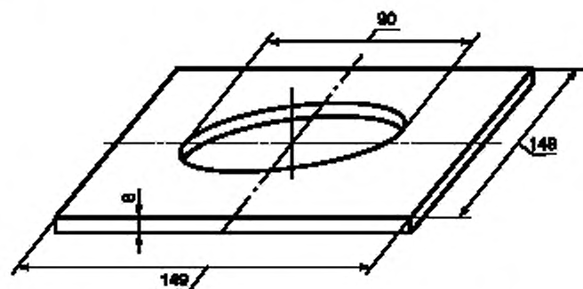
Рисунок 4 — Установочная пластина калориметра
