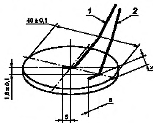
1 — константовый провод; 2 — медный провод
