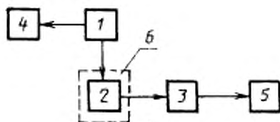
1—источник питания лавинного фотодиода; 2—испытываемый лавинный фотодиод; 3—операционный усилитель; 4—измеритель рабочего напряжения; 5—измеритель напряжения шума; 6—камера тепла и холода
