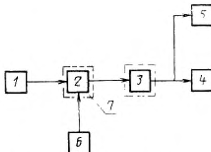
1—источник импульсного излучения, 2—испытываемый ФЭПП (ФПУ); 3—усилительное устройство; 4—регистрирующий прибор для измерения напряжения (тока) фотосигнала; 5—регистрирующий прибор для измерения напряжения (тока) шума; 6—источник питания; 7—камера тепла и холода
