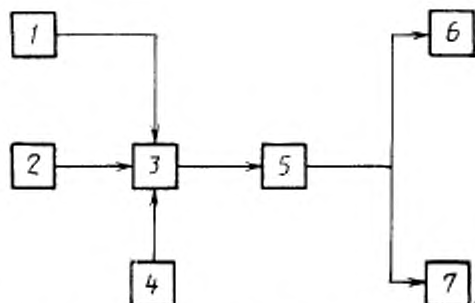
1—источник фонового излучения; 2—источник импульсного излучения; 3—испытуемый ФЭПП (ФПУ); 4—источник питания ФЭПП (ФПИ); 5—усилительное устройство; 6—регистрирующий прибор для измерения напряжения (тока) фотосигнала; 7—регистрирующий прибор для измерения напряжения (тока) шума
