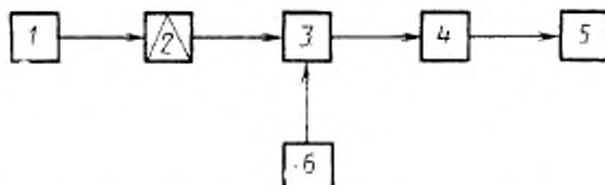
1—источник излучения; 2—модулятор; 3—испытуемый ФЭП (ФПУ); 4—усиливающее устройство; 5—регистрирующий прибор; 6—источник питания ФЭП (ФПУ).
