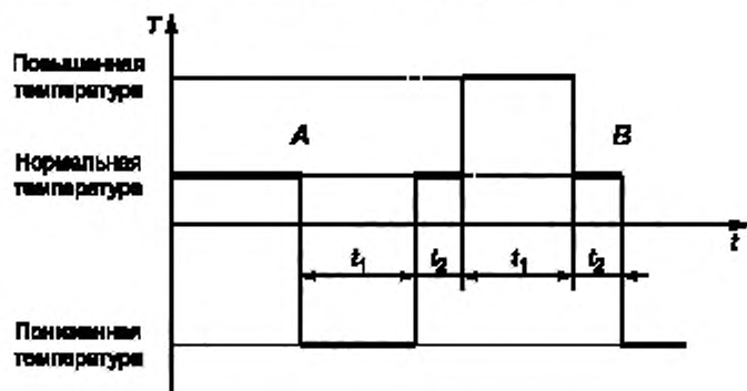
Рисунок 1 — График испытательного цикла
