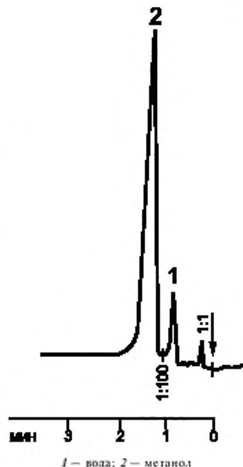
Рисунок Б.1 — Типовая хроматограмма технического метанола
