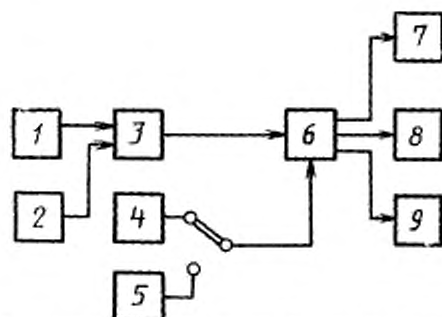
1 — основная оптическая система; 2 — дополнительная оптическая система; 3 — передающая трубка; 4 — генератор калиброванных прямоугольных импульсов (ГКИ); 5 — генератор калиброванных сигналов; 6 — видеоусилитель; 7 — видеоконтрольное устройство (ВКУ); 8 — осциллограф выделения строки (ОВС); 9 — измеритель шумов
