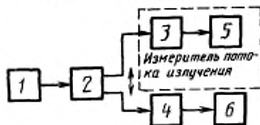
1 — осветитель; 2 — монохроматор; 3 — контрольный приемник излучения; 4 — передаточная трубка; 5 — измеритель фототока контрольного приемника; 6 — измеритель фототока фотокатода трубки.
