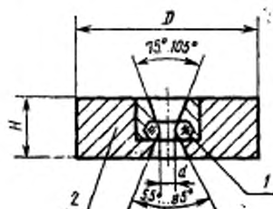
1 — алмаз; 2 — оправка; d — диаметр калибрующего отверстия
