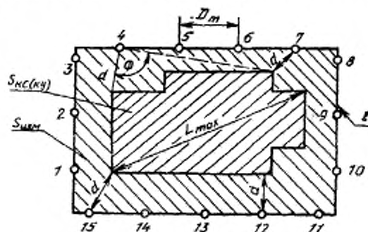
l — точки измерения; \Phi — угол обзора; D_{\text{из}} — расстояние между точками измерения; d — измерительное расстояние; L_{\text{из}}^{\text{из}} — наибольший размер по площади КС (КУ); S_{\text{из}}(\text{КУ}) — площадь КС (КУ); S_{\text{из}} — измерительная площадь; l — длина измерительного контура
