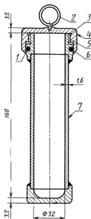
Испытательная бомба
