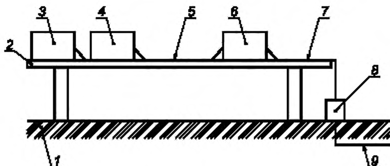
Рисунок 22 — Размещение блока питания при измерении излучаемых промышленных радиопомех в беззвонной камере (вид сбоку)
