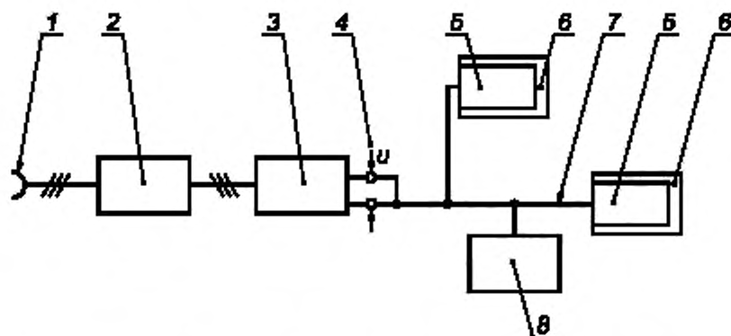
1 — сеть электропитания переменного тока 220 В, 50 Гц; 2 — испытательный генератор динамических изменений напряжения электропитания; 3 — испытываемый блок питания; 4 — напряжение на выходе блока питания, подаваемое в шину; 5 — передатчик/приемник; 6 — блок связи; 7 — кабель шины; 8 — устройство нагрузки шины
