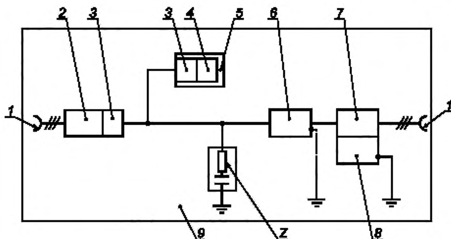
1 — сеть электропитания переменного тока 220 В, 50 Гц; 2 — блок питания, 3 — фильтр, 4 — передатчик/приемник; 5 — блок связи; 6 — испытательный блок, 7 — устройство связи/развязки; 8 — испытательный генератор МИП; 9 — непроводящая поверхность
