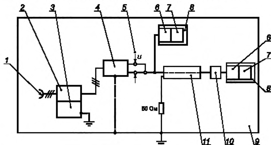
1 — сеть электропитания переменного тока 220 В, 50 Гц; 2 — устройство связи/развязки; 3 — испытательный генератор НИП; 4 — испытуемый блок питания; 5 — напряжение на выходе блока питания, подаваемое в шину; 6 — фильтр; 7 — передатчик/приемник; 8 — блок связи; 9 — пластина заземления; 10 — аттенюатор; 11 — емкостные клещи связи
