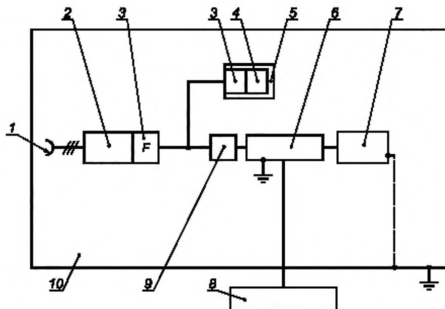
1 — сеть электропитания переменного тока 220 В, 50 Гц; 2 — блок питания; 3 — фильтр; 4 — передатчик/приемник; 5 — блок связи; 6 — устройство связи/развязки; 7 — испытываемое устройство; 8 — генератор сигналов высокой частоты и усилитель; 9 — аттенюатор; 10 — пластина заземления
