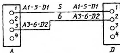
Черт. 7. Пример сложной маркировки для двух проводов
