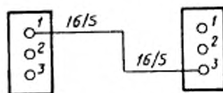
Черт. 13. Независимая маркировка
