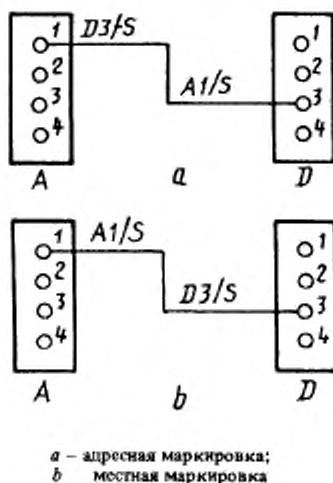
Черт. 11. Примеры зависимой маркировки с дополнительной маркировкой
