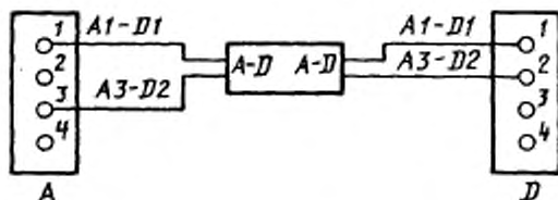
Черт. 2. Пример зависимой двойной маркировки для двух проводов и группы проводов (кабеля)
