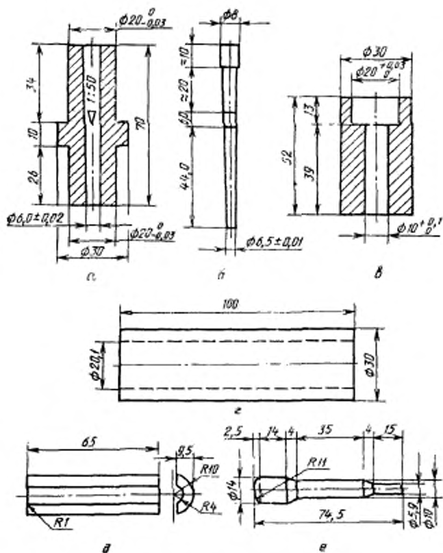
а — форма; б — калибр; в — направляющая выталкивающего устройства; г — направляющая трубка; д — приемник; е — выталкивающий поршень
