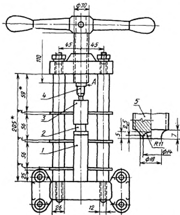
1 — трубка направляющего устройства; 2 — форма; 3 — направляющее устройство; 4 — выталкивающий поршень; 5 — конец штыря А
