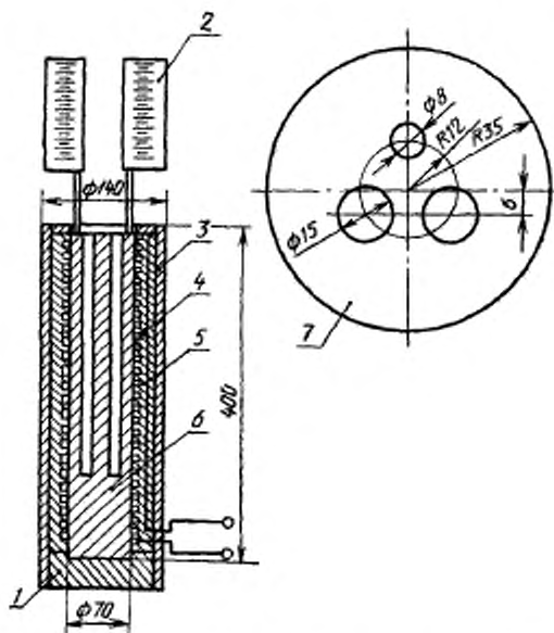
1 — огнеупорный материал; 2 — зеркало; 3 — асбестосемент; 4 — ил; 5 — смесь магния и асбеста; 6 — алюминиевая бронза; 7 — положение отверстий
