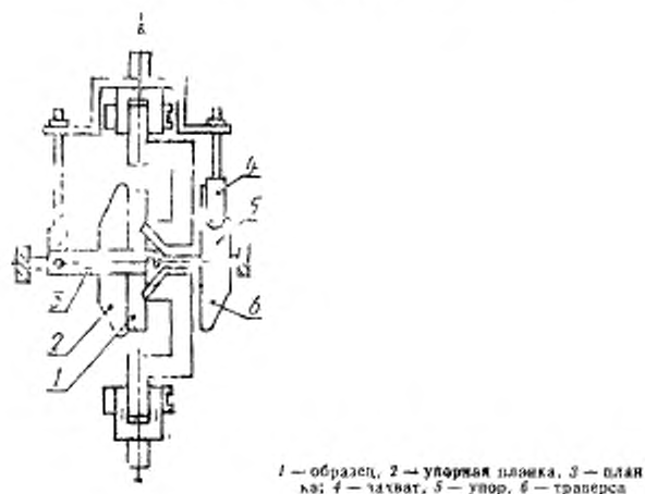
Черт. 1
