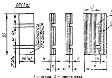
Черт. 3
