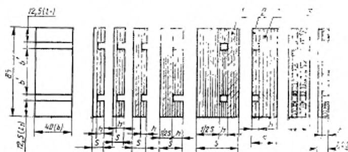
Черт. 2, лист 2
