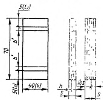
Черт. 2, лист 1
