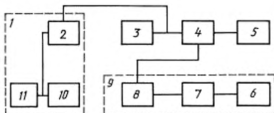
1, 9 — экранированная камера; 2 — устройство регулируемой связи; 3 — контролируемый ГППП СВЧ; 4 — направленный ответвитель; 5, 11 — согласованная нагрузка; 6 — измерительное устройство (приемник); 7 — аттенуатор; 8 — фильтр; 10 — дополнительный генератор
