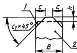
Смежные зубья
