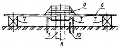
Установка комбинированная
