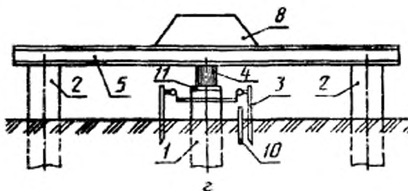
Установка комбинированная
