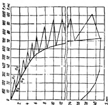
Рисунок 1 — График зависимости остатков strain S от нагрузки P
