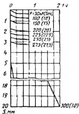
График изменения осадки свая S во времени t (по ступеням нагружения)
