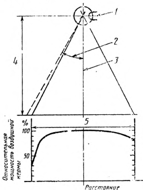
1 — ФОКУСНОЕ ПЯТНО; 2 — УГОЛ НАКЛОНА ЗЕРКАЛА К ОСИ АНОДА; 3 — ОПОРНАЯ ОСЬ; 4 — нормированное расстояние; 5 — нормированное максимальное симметричное РАДИАЦИОННОЕ ПОЛЕ
