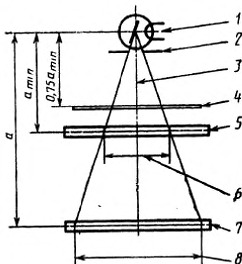
1 — ФОКУСНОЕ ПЯТНО; 2 — ДИАФРАГМА; 3 — ОПОРНАЯ ОСЬ; 4 — ДОПОЛНИТЕЛЬНЫЙ ФИЛЬТР по таблице 1; 5 — плоскость измерения на расстоянии a_{\min} ; 6 — РАДИАЦИОННОЕ ПОЛЕ на расстоянии a_{\min} ; 7 — плоскость измерения на расстоянии a ; 8 — РАДИАЦИОННОЕ ПОЛЕ на расстоянии a
