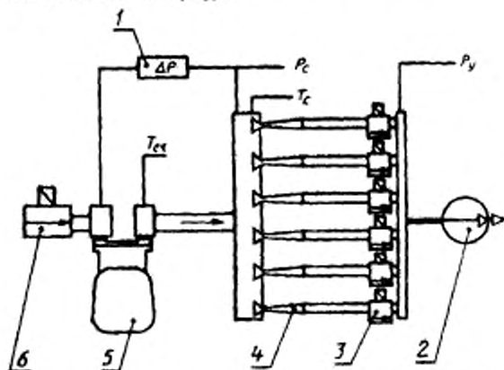
1 — дифманометр измерения потери давления \Delta P на счетчике; 2 — вакуумный насос; 3 — выходные краны сопел; 4 — образцовое звуковое сопло; 5 — испытуемый счетчик; 6 — входной кран установки; T_{с\kappa} — температура на выходе испытуемого счетчика; T_c — температура на входе сопла; P_c — давление на входе сопла; P_y — давление на выходе сопла
