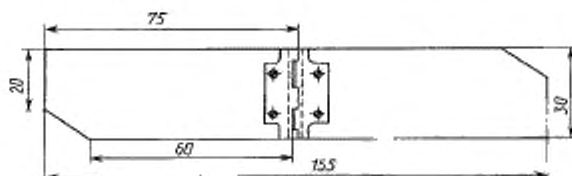
Рисунок 2 — Давильная пластинка
