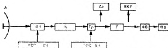
Рисунок 8 — Структурная схема измерений «статистического порога» отношения сигнал/шум и энергетического потенциала приемной установки
