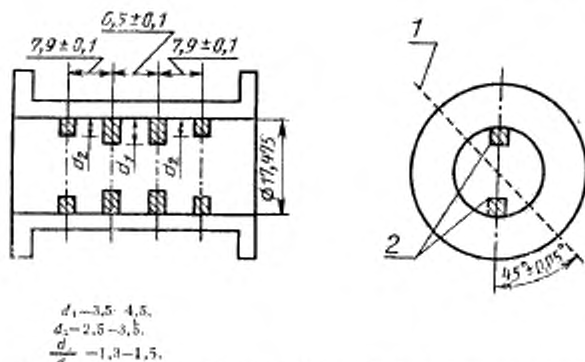
1 — электрическое поле на входе прямоугольного волновода; 2 — винты М3 Рисунок В4 — Основные размеры круглого поляризатора
