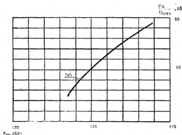
Рисунок 9 Тилловая зависимость напряжения шума от мощности входного высокочастотного сигнала или сигнала промежуточной частоты.
