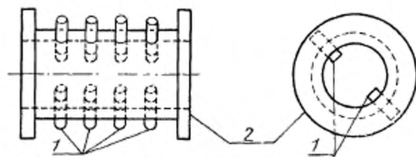
1 — подстроечные винты; 2 — круглый волновод
