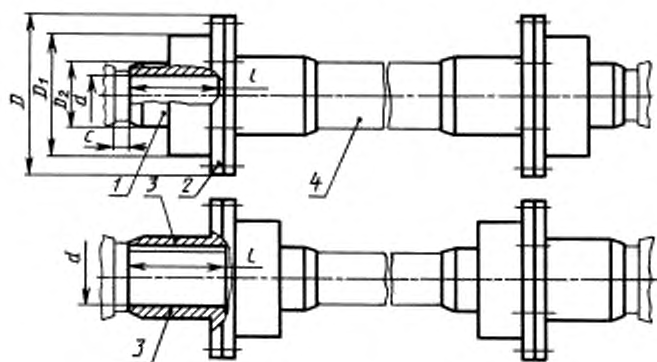
Варианты сборки
