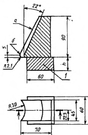
1 — три пластины: h = 25,6 мм; h = 27,6 мм; h = 29,6 мм. а — конус (концентричен с цилиндром); б — цилиндр
