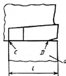
Тип А: l = 100 мм. Тип С: l = 80 мм. a — испытательная плоскость
