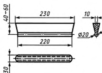
Рисунок 4 — Заготовка для вырезки образцов
