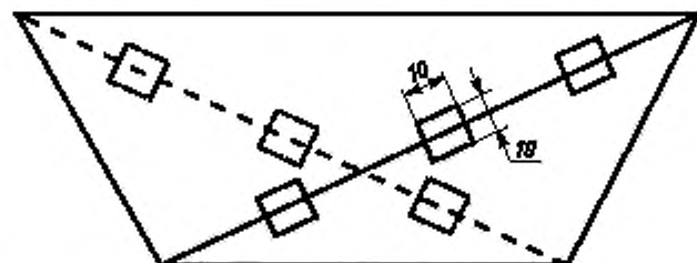
Рисунок Б.2 — Схема расположения квадратов на макрошлифе
