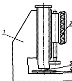
1 — корпус; 2 — индикатор часового типа; 3 — индентор; 4 — образец
