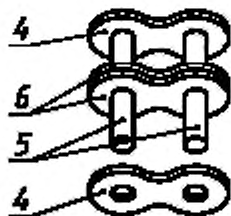
в — наружное звено двухкорданное
