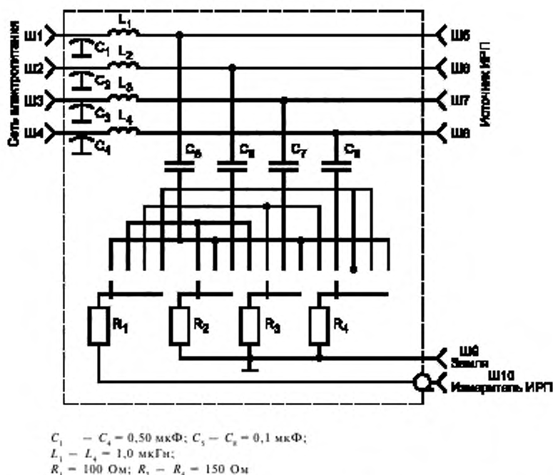
Рисунок Г.2 — Принципиальная схема четырехфазного V-образного эквивалента сети типа 2
