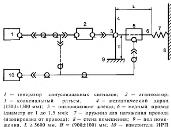
Рисунок 8 — Схема проверки погрешности коэффициента калибровки поглощающих клещей
