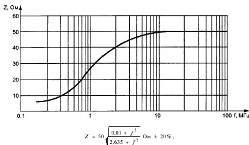
Рисунок 6 — Модуль полного входного сопротивления V-образного эквивалента сети типа 5 (50 Ом/5 мкГц + 1 Ом)
