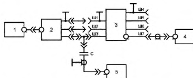
1 — согласованная нагрузка; 2 — испытуемый измеритель ИРП; 3 — V-образный эквивалент сети типов 1, 2, 4, 5; 4 — дополнительный измеритель ИРП; 5 — генератор синусоидальных сигналов; C — 0,1 мкФ ±20 % — разделительный конденсатор; Ш1, Ш4 — разъемы «ЗЕМЛЯ»; Ш2, Ш3 — разъемы «ИСТОЧНИК ИРП»; Ш5, Ш6 — разъемы «СЕТЬ ЭЛЕКТРОПИТАНИЯ»; Ш7 — разъем «ИЗМЕРИТЕЛЬ ИРП».
