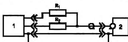
1 — измеритель ИРП; 2 — генератор синусоидальных сигналов; R_1 = R_2 = (300 \pm 1) \text{ Ом}
