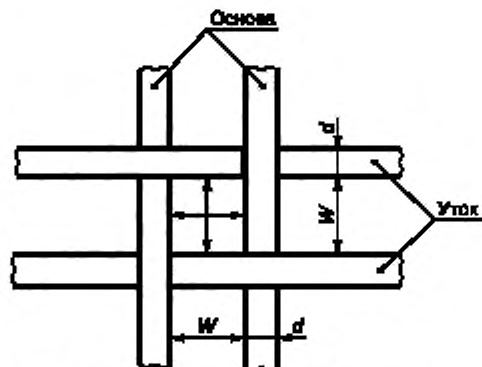
Рисунок 1 — Ячейка сетки
