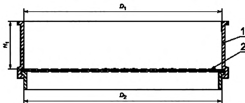
1 — обечайка (рамка); 2 — сетка из металлической проволоки
