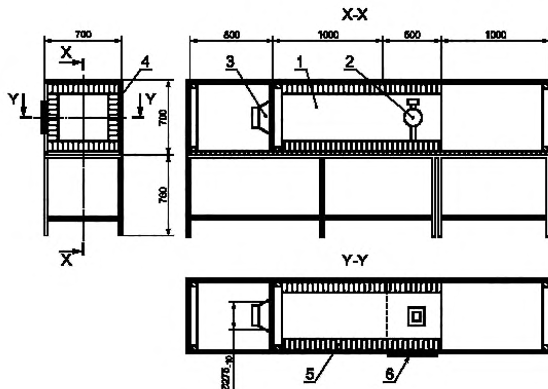
1 — акустический тоннель, 2 — устройство для установки образцов; 3 — динамик; 4 — стенки тоннеля (из деревянной доски толщиной 17 мм); 5 — изолирующие блоки из стеклоблоков (толщиной 100 мм); 6 — дверь
