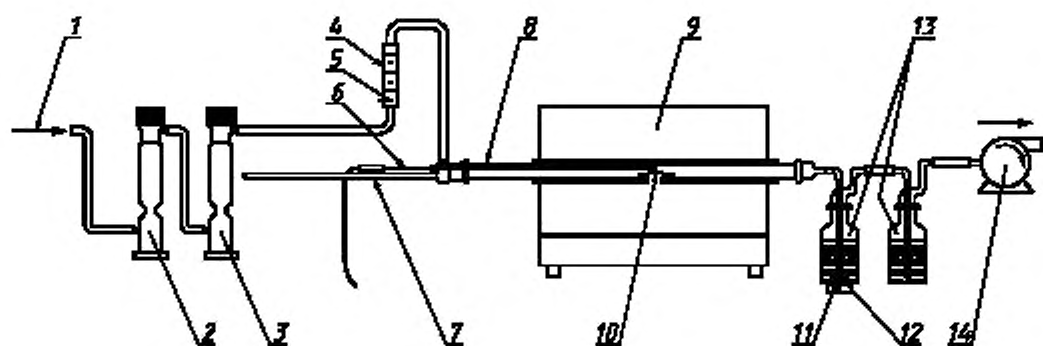
1 — воздух окружающей среды; 2 — воздушный фильтр (активированный уголь); 3 — осушитель воздуха (селикатель); 4 — ротаметр; 5 — игольчатый вентиль; 6 — термопара; 7 — устройство для ввода лодочки с образцом; 8 — трубка из кварцевого стекла; 9 — печь; 10 — лодочка с образцом; 11 — магнитная мешалка; 12 — стержень магнитной мешалки; 13 — промывочные сосуды; 14 — всасывающий насос
