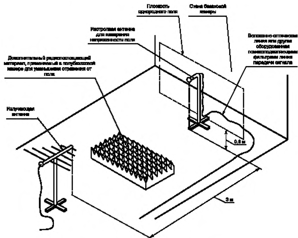
Рисунок 3 — Расположение оборудования при аттестации
