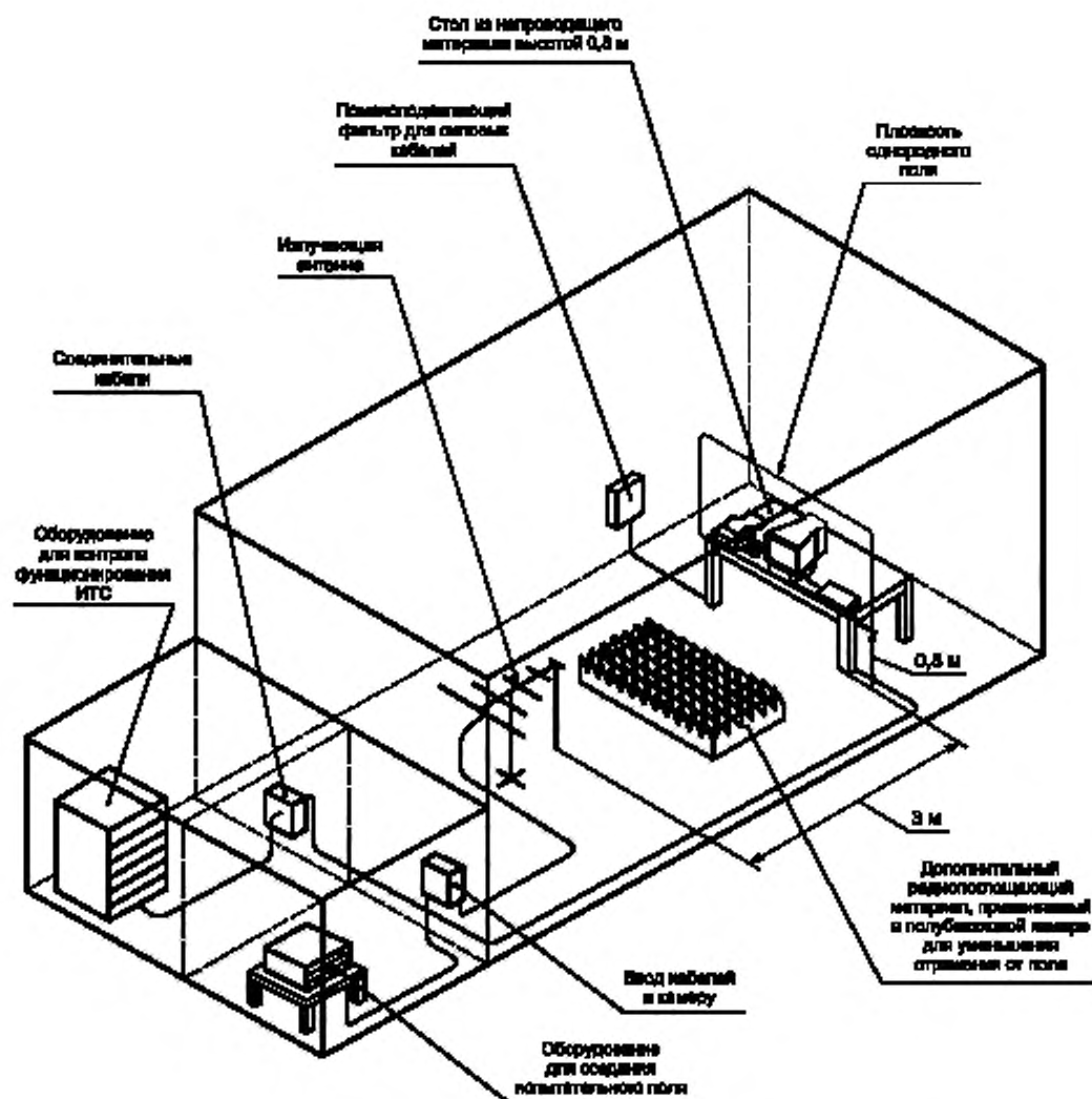
Рисунок 2 — Пример средств испытаний, удовлетворяющих требованиям стандарта
