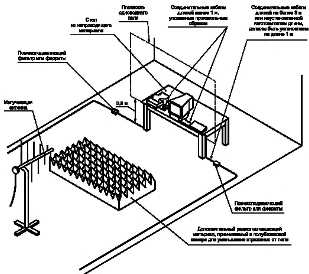
Рисунок 6 — Пример рабочего места для испытаний настольных ТС
