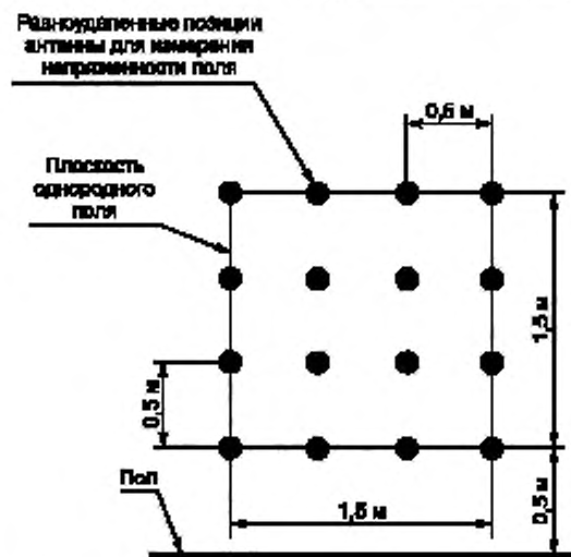
Рисунок 4 — Размеры плоскости однородного поля
