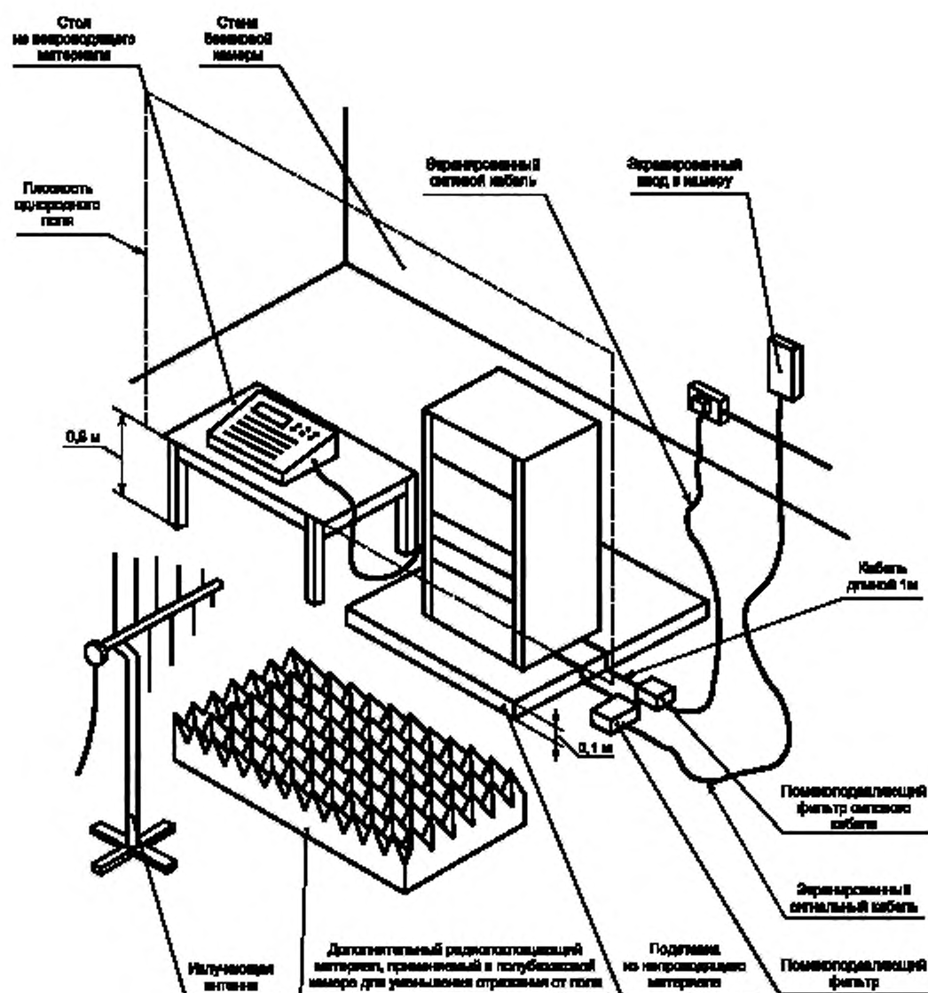
Рисунок 5 — Пример рабочего места для испытаний напольных ТС
