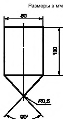
Рисунок 6 — Испытательный конус
