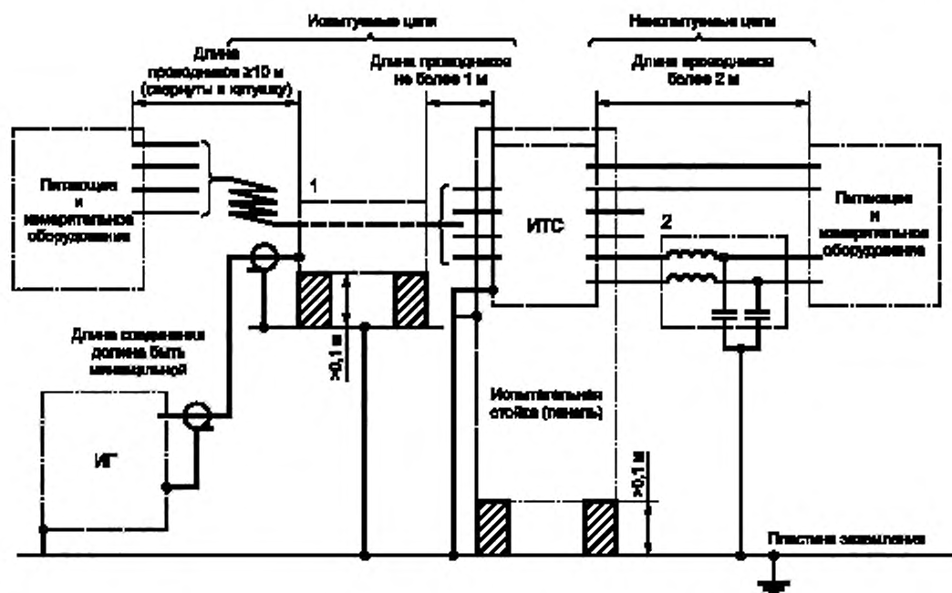
1 — емкостные клещи связи; 2 — фильтр развязки (применяется при необходимости)
