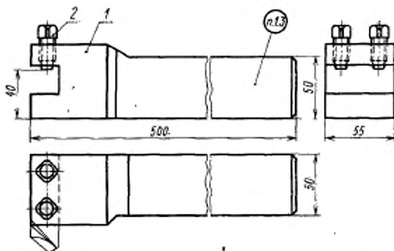
1—корпус; 2—винт В.М12—6g×25.33Н.05 ГОСТ 1482—84 Черт. 1
