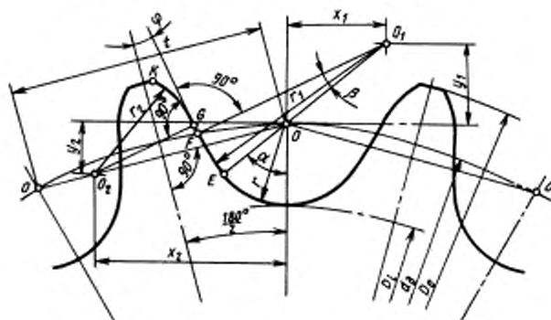
Профиль зубьев без смещения центров дуг впадин
