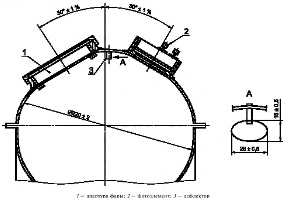
Рисунок А.1 — Схема светомерного (Ulbricht) шара
