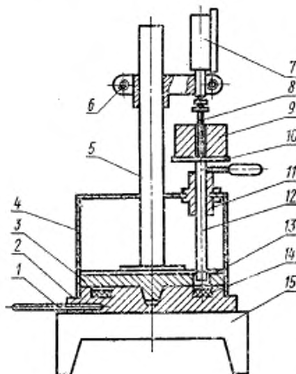
1—термометр; 2—нижняя плита; 3—верхняя плита; 4—кожух; 5—стойка; 6—держатель индикаторов; 7—индикатор; 8—узел индикатора; 9—груз; 10—площадка груза; 11—направляющая игла; 12—шток; 13—пуансон; 14—образец; 15—нагреватель.
