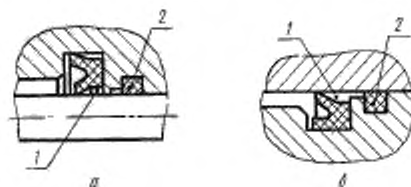
1 — место закладки смазки, 2 — войлочное кольцо.
